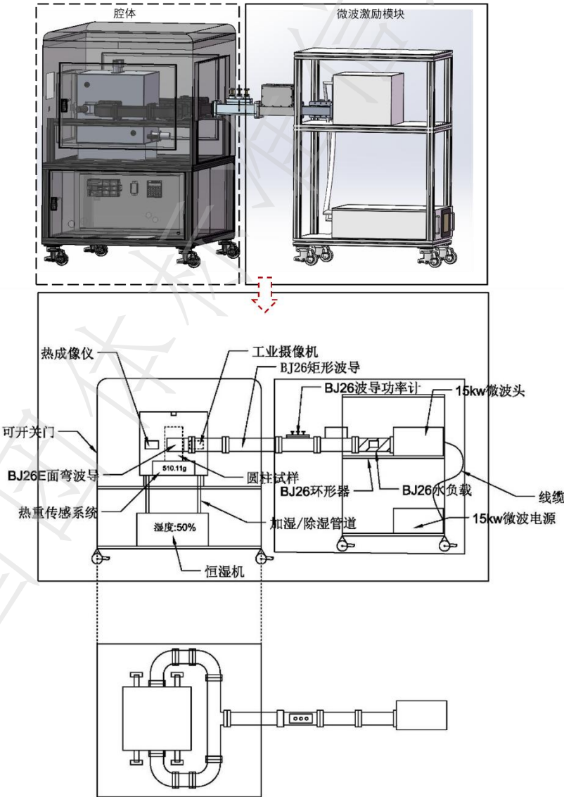
图 1 微波作用腔体
