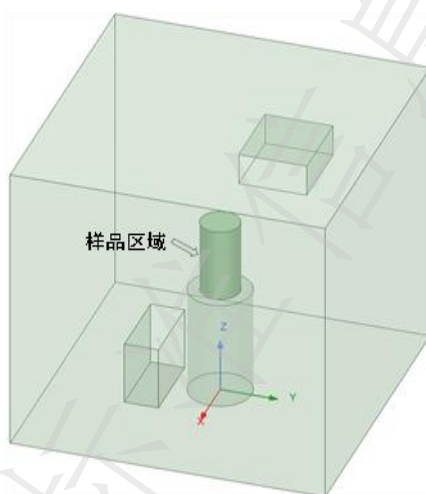
图 2 微波致裂试验示意图
